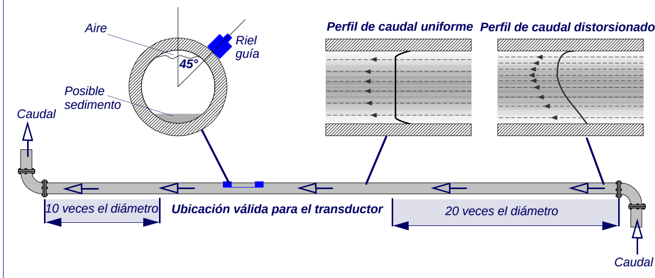
Figura 2.1 Ubicación de los transductores
