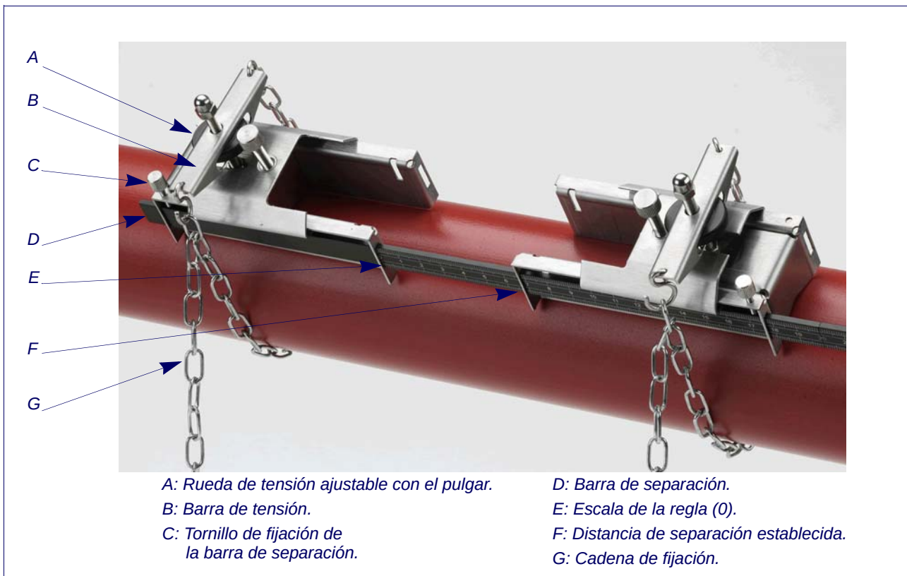
Figura 2.2 Montaje del riel guía
