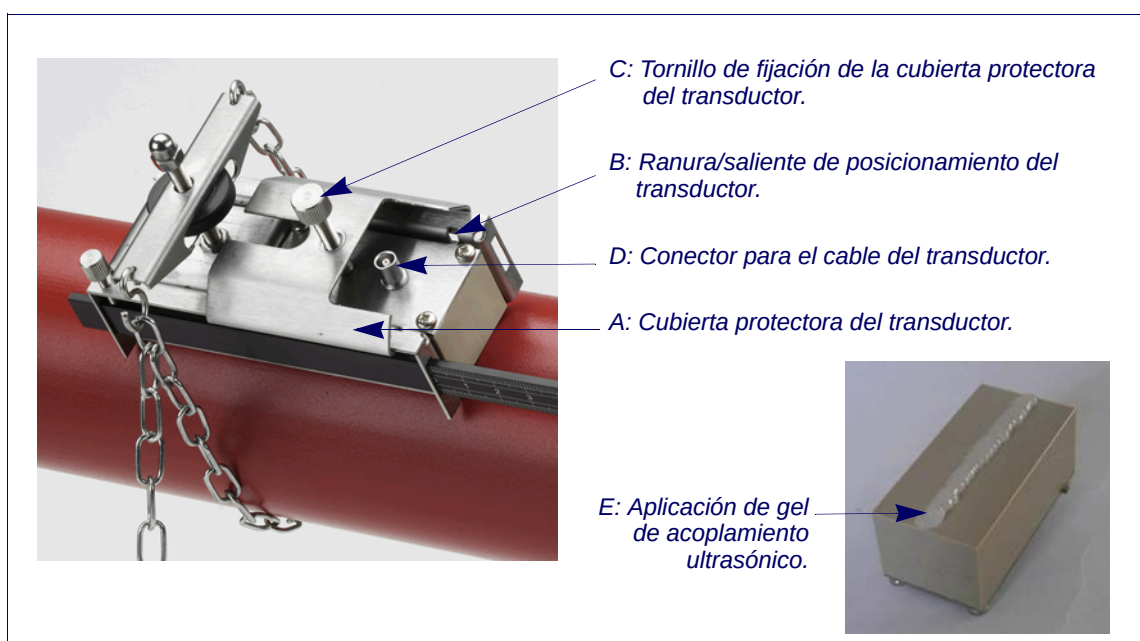
Figura 2.3 Montaje de los transductores
